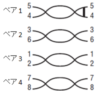
図 4-9 短絡(ショート):ペア内
