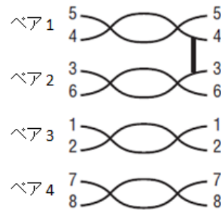
図 4-10 短絡(ショート):ペア間
