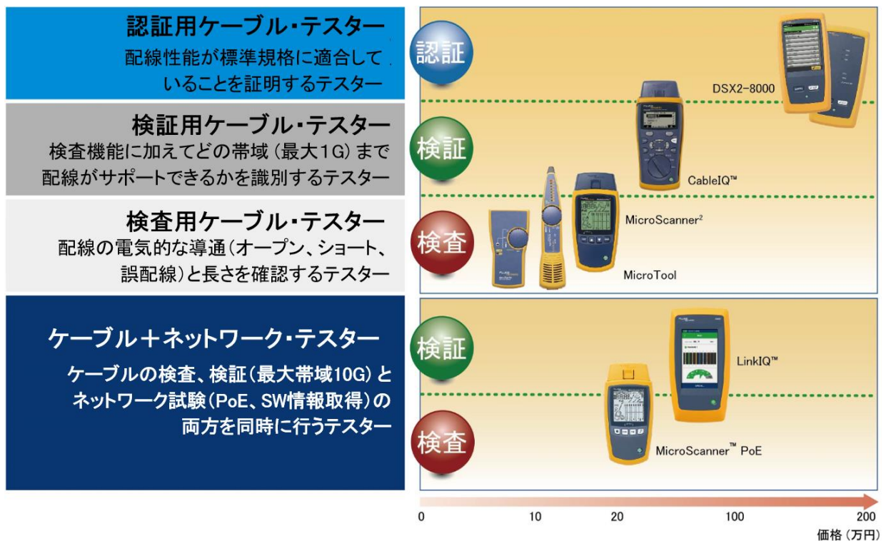
図 5-1 ケーブル・テスターの種類
