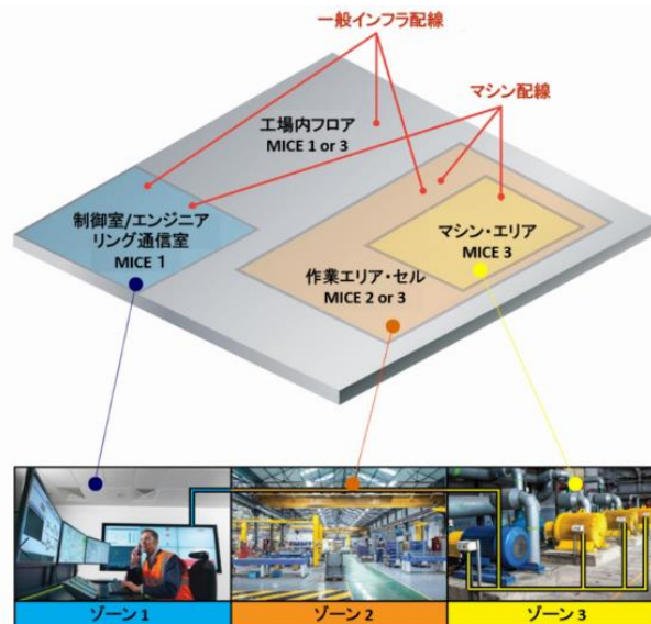
図 5-7 MICE 環境のクラスとゾーン
