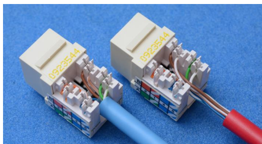
写真 4-4 撚り戻しは最小限にする
