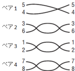
図 4-11 対反転(リバースペア)
