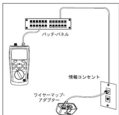
図 6-10 標準のワイヤー・マップ・アダプターを使用することで情報コンセントまでの接続性試験例
