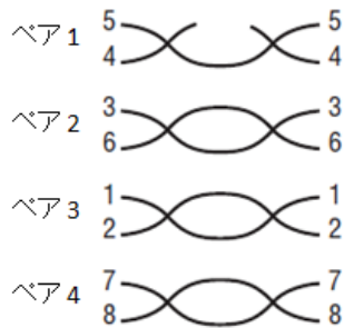
図 4-8 開放(オープン)
