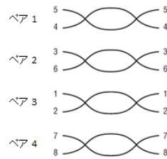
図 4-7 ワイヤー・マップが正しい組合せの場合
