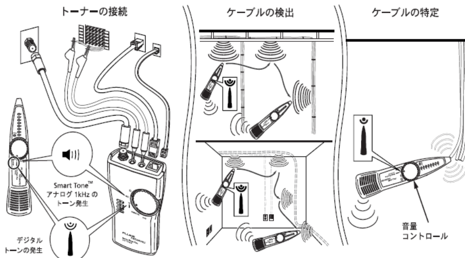
図 6-32 IntelliTone トナー & プローブを壁裏やドロップ配線の識別・検知での使用
