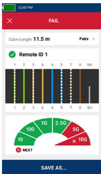
図 6-20 ケーブル試験の不合格結果
