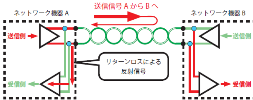
図 4-17 リターンロス
