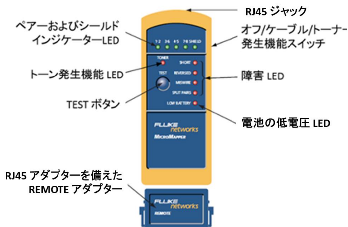
図 6-28 MicroMapper の本体パネル LED 表示とリモート・アダプター
