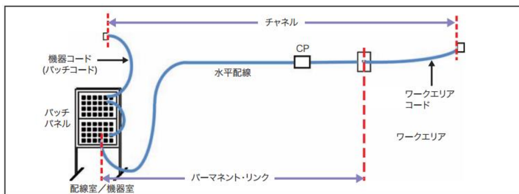
図 4-6 LAN 配線の構成(パーマネント・リンクとチャネル)
