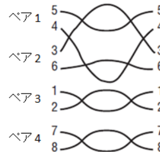
図 4-13 対分割(スプリットペア)
