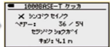
図 6-7 詳細情報の表示例
