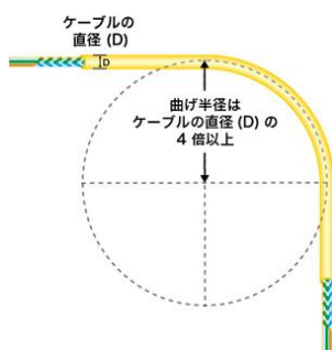
図 4-4 ケーブルの曲げ半径
