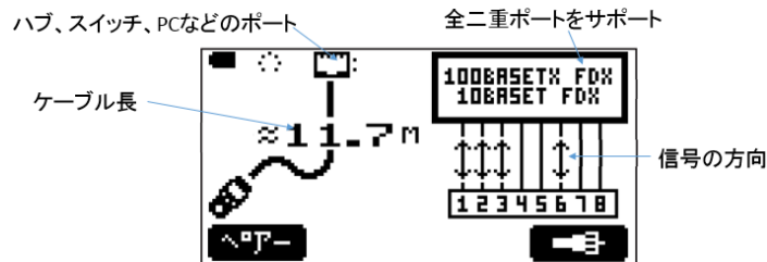
図 6-8 検知モードの結果画面表示例
