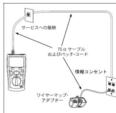
図 6-12 標準のワイヤー・マップ・アダプターを使用した同軸ケーブルの接続性試験例
