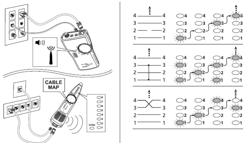
図 6-33 ワイヤー・マップ試験結果表示例
