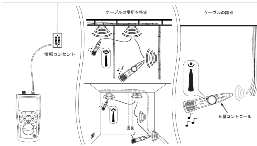
図 6-14 トーン・プローブを使ったケーブルのトレース使用例
