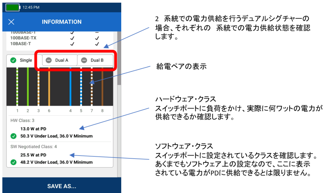
図 6-24 PoE 試験結果
