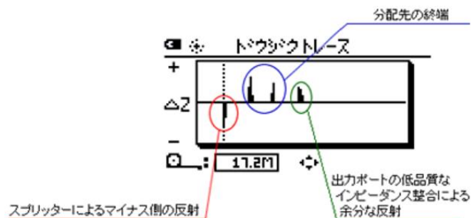
図 6-13 同軸ケーブルの TDR プロット図表示例
