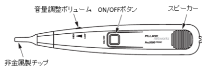
図 6-34 Pro3000 プローブ
