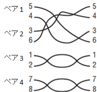
図 4-12 対間交差(クロスペア)
