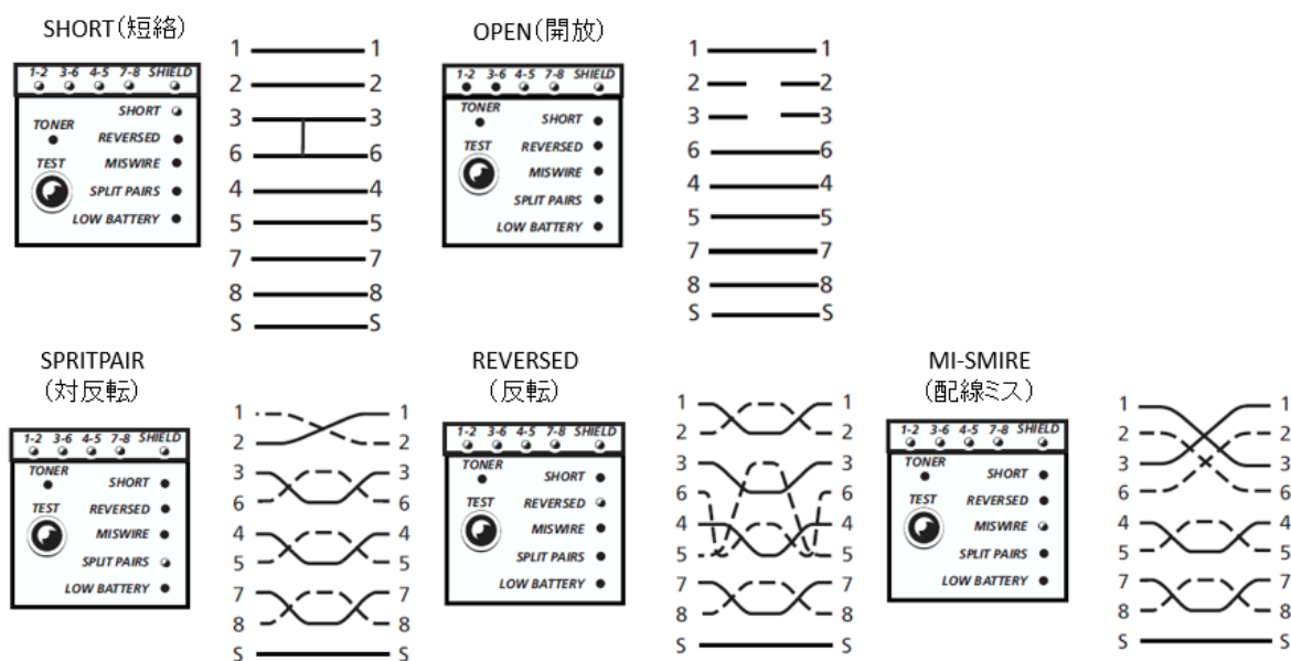
図 6-29 MicroMapper のワイヤー・マップ結果 LED 表示
