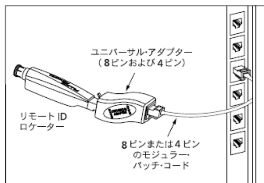
図 6-11 オプションのリモート ID ロケーターを使用してパッチパネルの接続性と配線のワイヤー・マップ試験例
