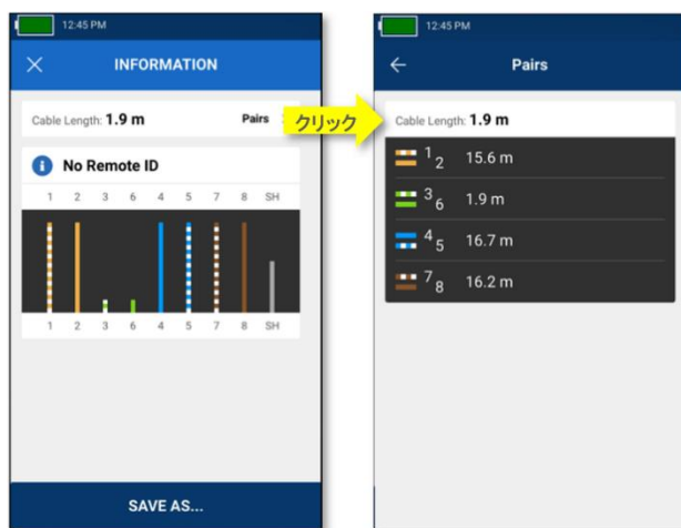
図 6-21 ケーブル試験の不合格結果
