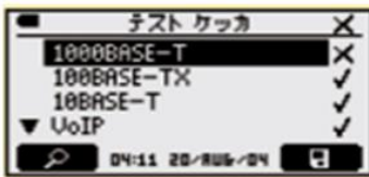
図 6-5 オートテスト結果不合格例
