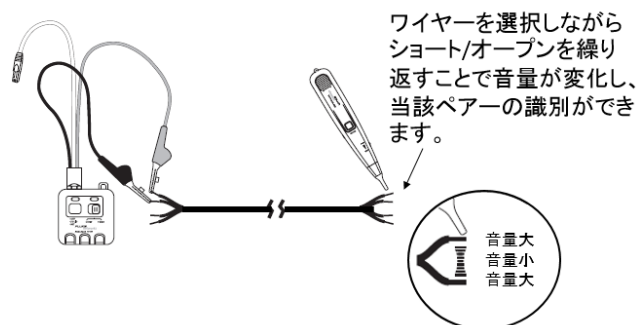
図 6-36 SmartTone®機能による各ペアの識別使用例
