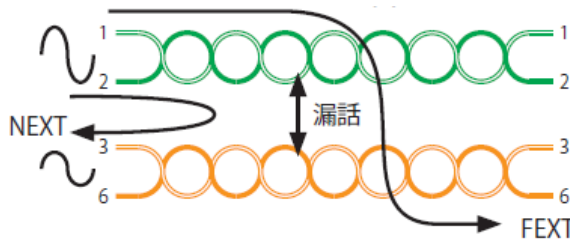
図 4-16 漏話(NEXT)
